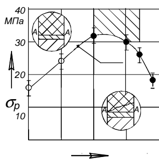
Рис. 2. Зависимость механической прочности сварного соединения ТВ-2 +ХН67ВМТЮ от толщины барьерной прослойки хрома (при T=1074 К; P=15 МПа, V \leq 1,3 \cdot 10 Па, t = 300 с);
