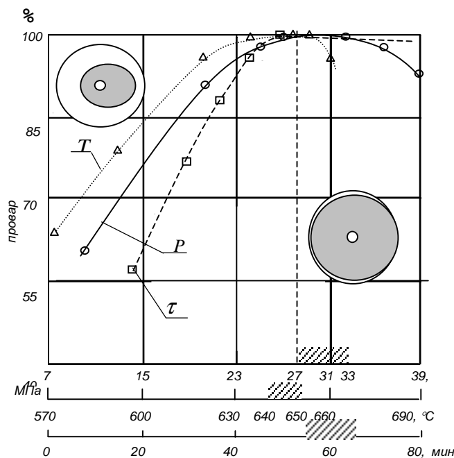
Рис. 5. Зависимость поверхности разрушения сварного соединения по пьезокерамике от режима сварки. P - усилие сжатия, T – температура сварки, τ - время сварки.
