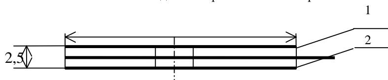
Рис. 4. Металлопьезокерамический биморф. 1 – пьезокерамика; 2 – титановый электрод.
