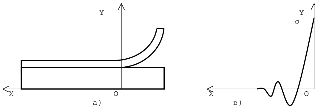
Рис 3. а) разрушение слоистой конструкции; в) распределение нормальных напряжений на границе металл-пьезокерамика, О – точка начала расслоения.
